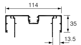
Door Frame CI-3220 (CI-7602)
