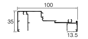
Window Sill CI-2250 (CI-6405)
