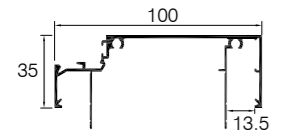
Offset Sill CI-2253 (CI-6435)
