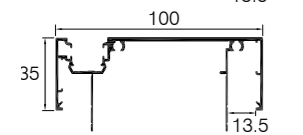
Offset Frame CI-2233 (CI-6432)
