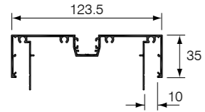
Door Frame CI-4920 (CI-9102)
