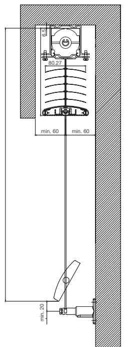
CABLE GUIDE
