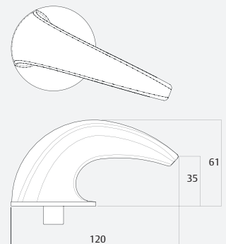
Lever 23
