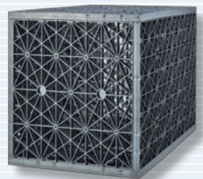
Flo-Tank® module
